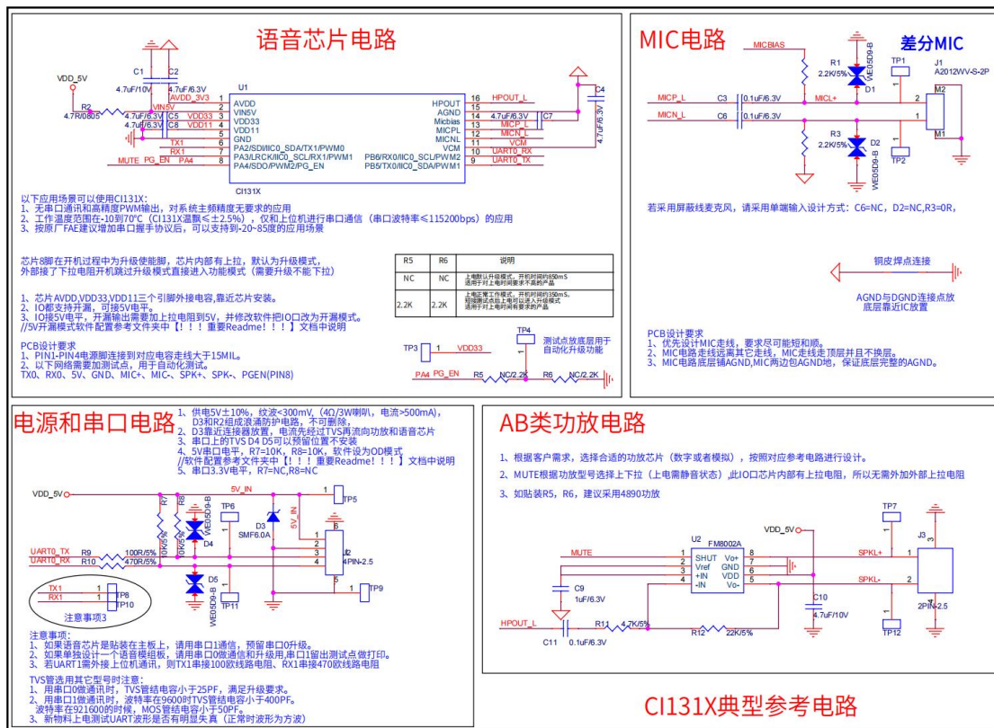
图 11: CI131X 典型方案的应用参考电路图
