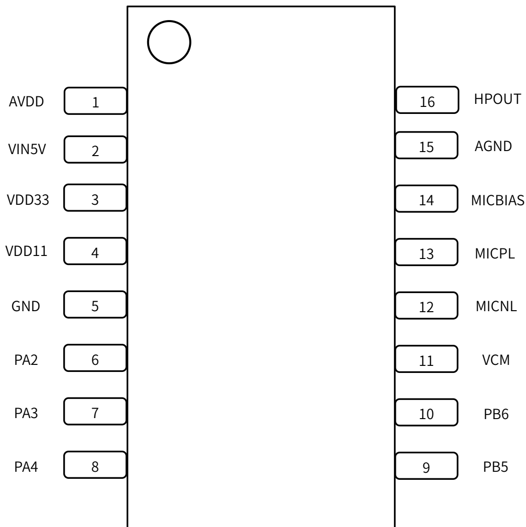
图 2: SOP16 引脚图
