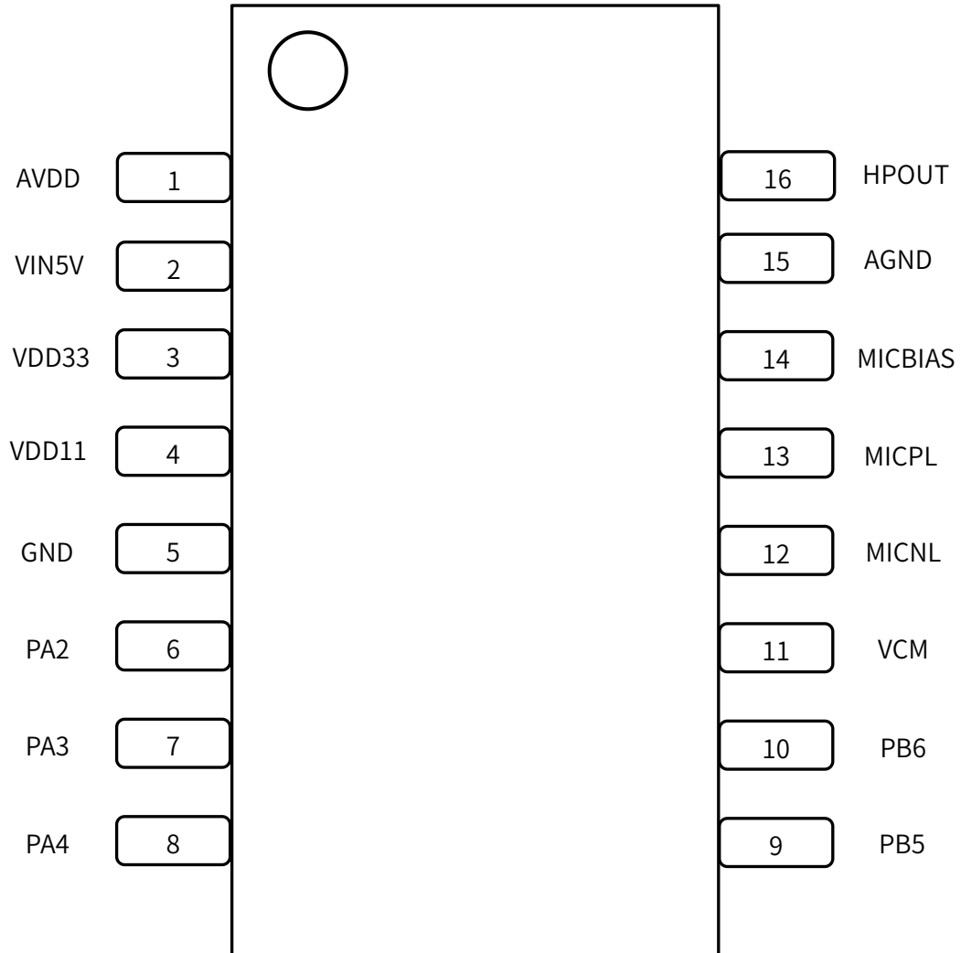
图 2: SOP16 引脚图
