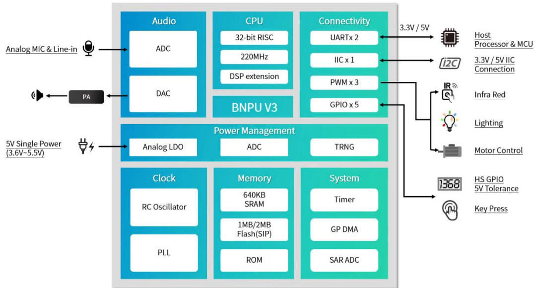
图 1：芯片功能框图
