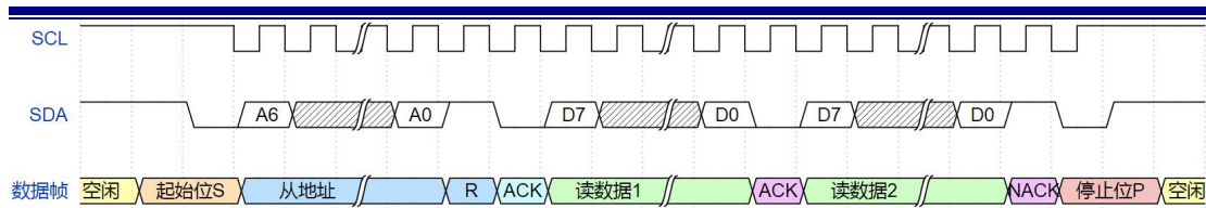
图 9: IIC 读操作时序图
