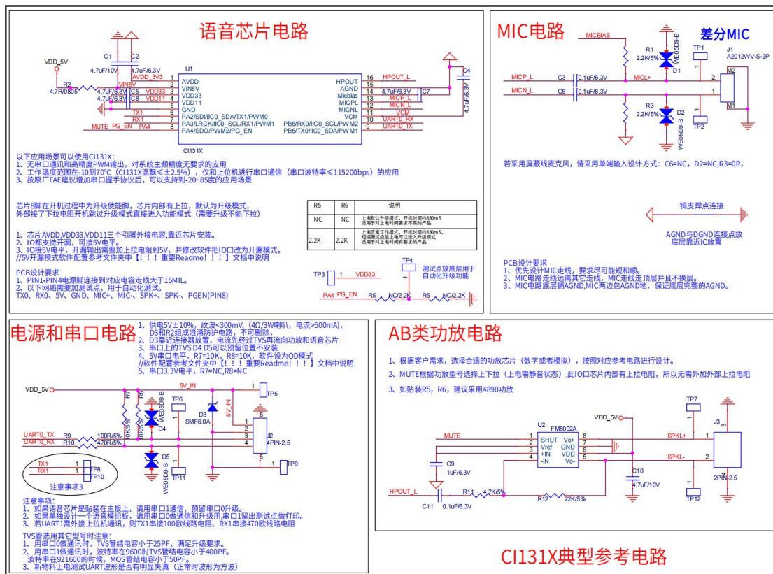
图 11: CI131X 典型应用方案参考电路图
