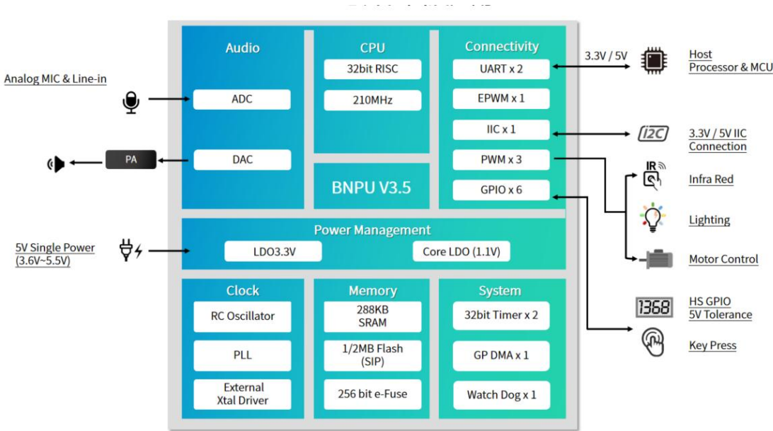
图 1： CI13161 功能框图
