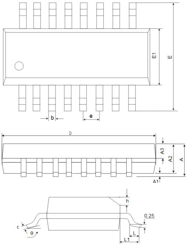
图 10：封装尺寸
