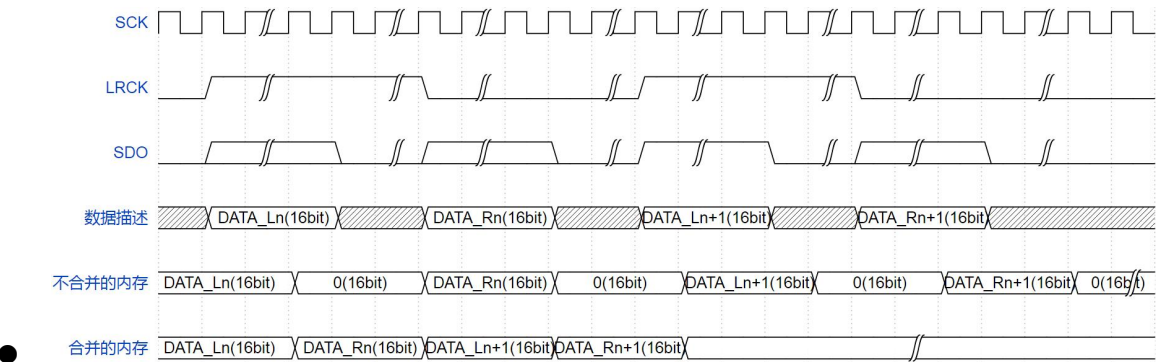
图 6：声道合并功能原理图
