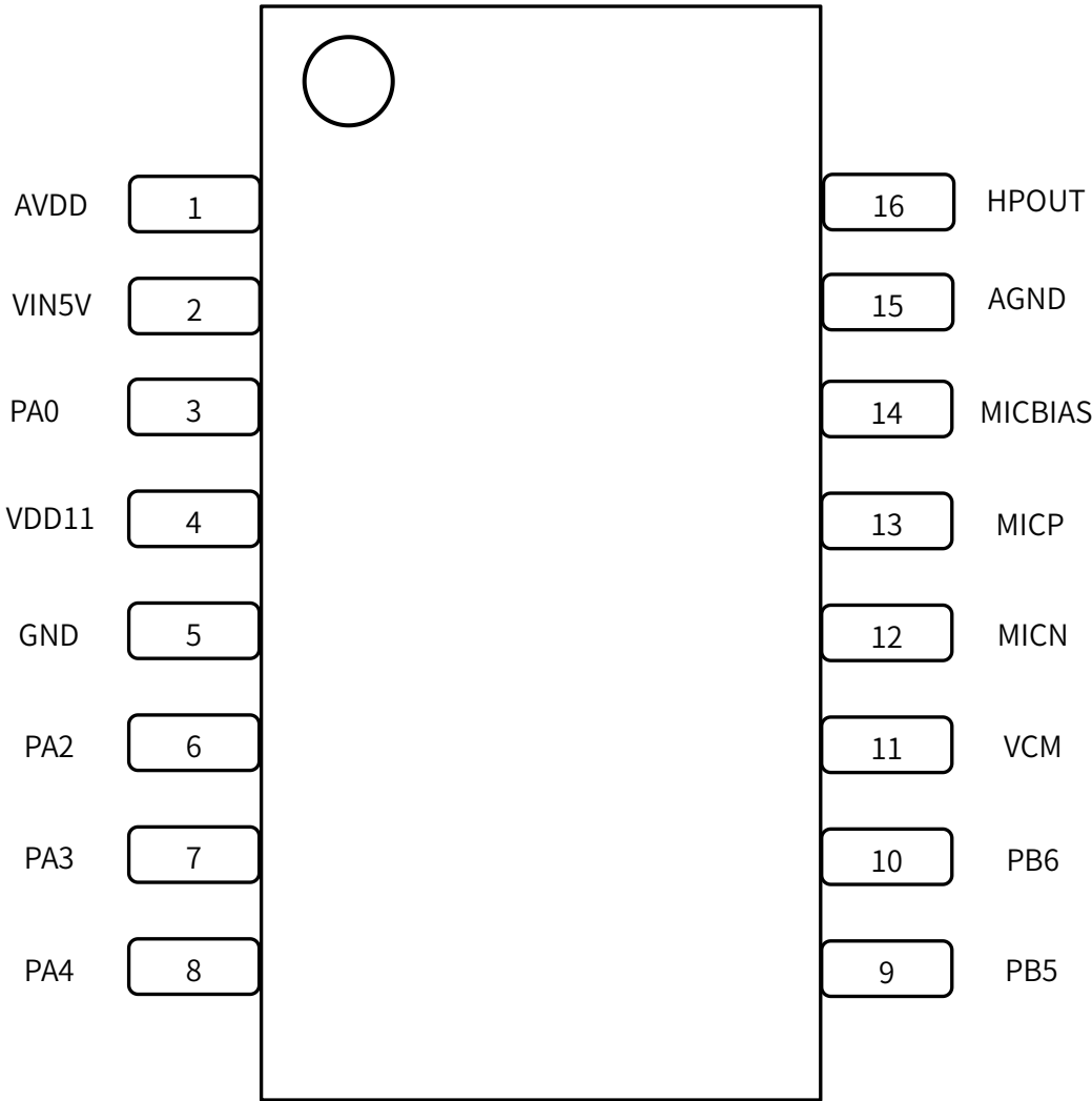
图 2： CI13162 管脚顺序及定义图
