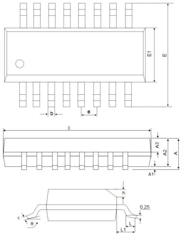
图 10：封装尺寸
