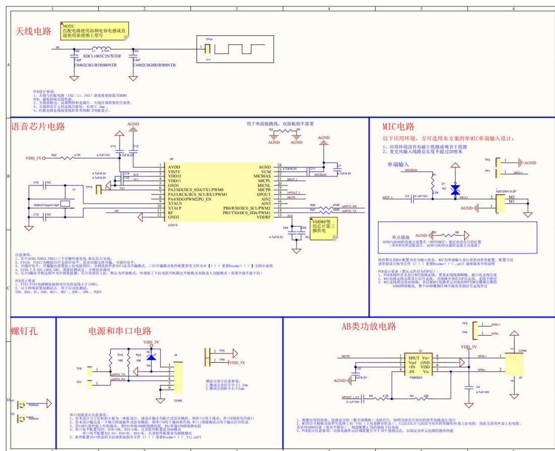
图 6-1 CI2311 方案的应用参考电路图
