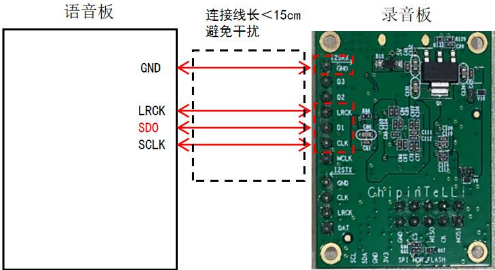
语音板与采音板连接框图
