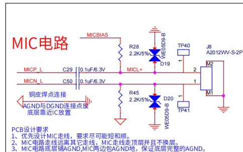
图 9 麦克风的差分线路
