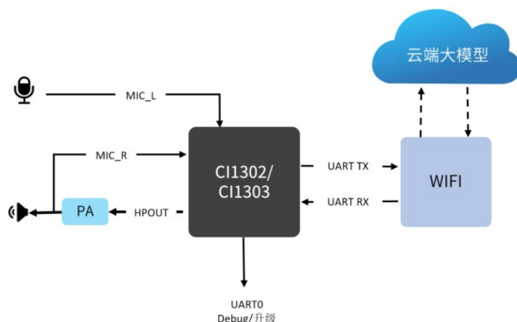
图 1 CI130X+wifi 离在线大模型方案框图
