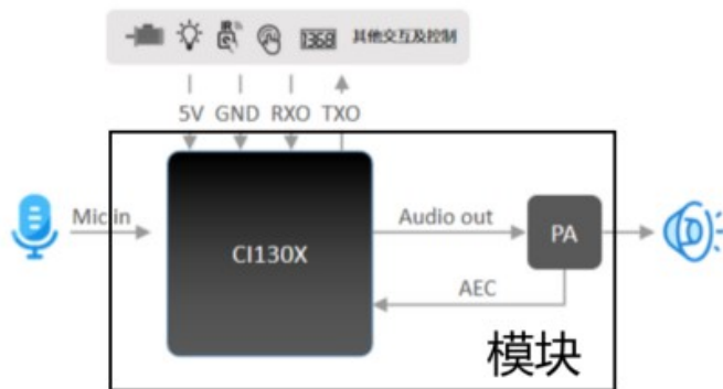
图 4 D02GS01J 的模块板示意图
