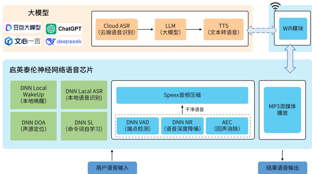
图 2 130X 软件功能框图
