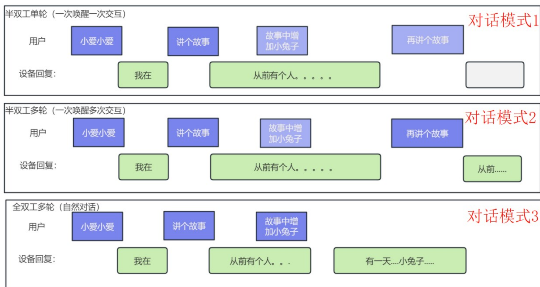
图 3：多种对话模式：模式 1 半双工单轮对话，模式 2 半双工多轮，模式 3 全双工多轮自然对话
