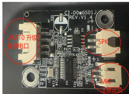
图 5b、D02GS01J 模块板正面
