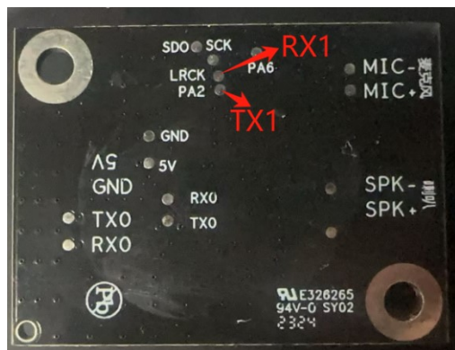
图 5a D02GS01J 模块板反面
